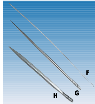
F/797 504 .. Längen / lengths: 8, 9, 10 cm / 3, 3.6, 4 inches Stahlborste VE 25 Stück Steel bristle pack. unit 50 pieces G/797 012 .. Größen / sizes: 50, 60, 70, 80 mm / 2.0, 2.4, 2.8, 3.2 inches Stappahle rund Spitze / Awl round G/797 012 .. Größen / sizes: 50, 60, 70, 80 mm / 2.0, 2.4, 2.8, 3.2 inches Stappahle rund Spitze / Awl round
